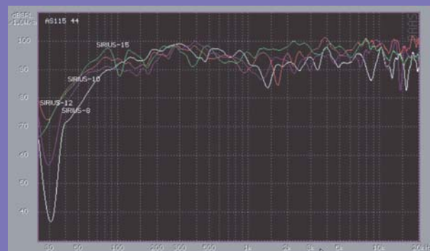
Courbe de réponse des fréquences Frequency responses
